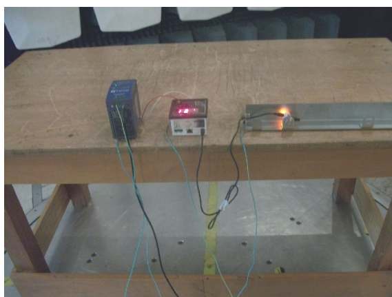
Fotos 12 e 13 – Emissão de perturbação radiada
