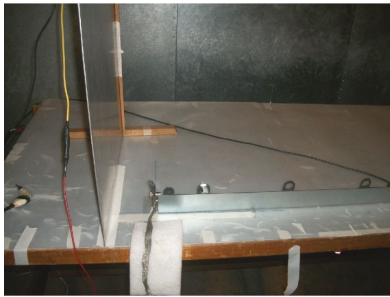
Foto 22: Vista traseira horizontal e direita vertical do ESE.
