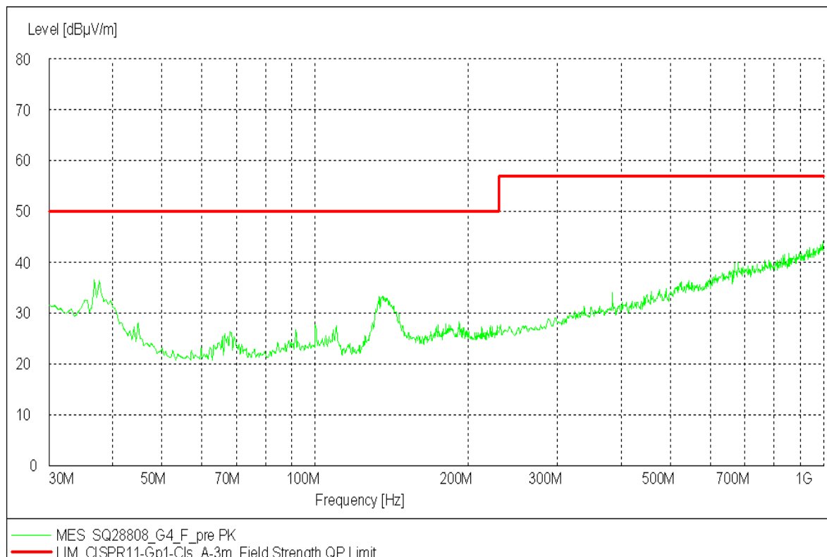
Gráfico 1 - Resultados do Ensaio de Emissão de Perturbação Radiada – Configuração Padrão - Alimentação 220V @ 60 Hz (24Vcc output) – Amostra 5284
