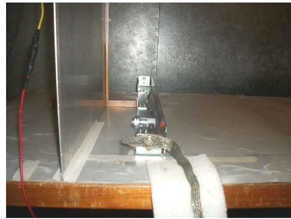
Foto 23: Vista esquerda horizontal e traseira vertical do ESE.
