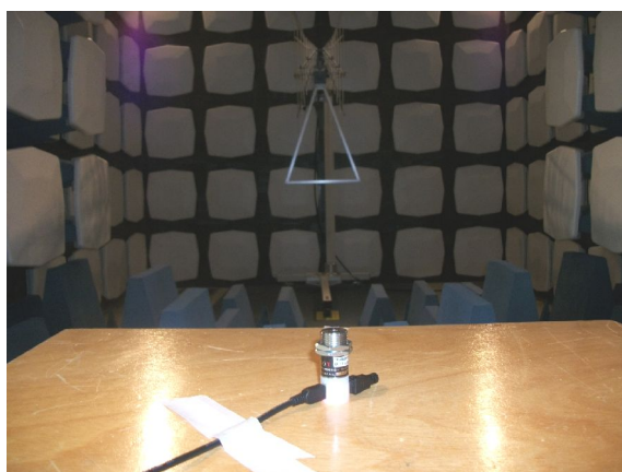
Fotos 14 e 15 – Imunidade a Radiofrequência irradiada
