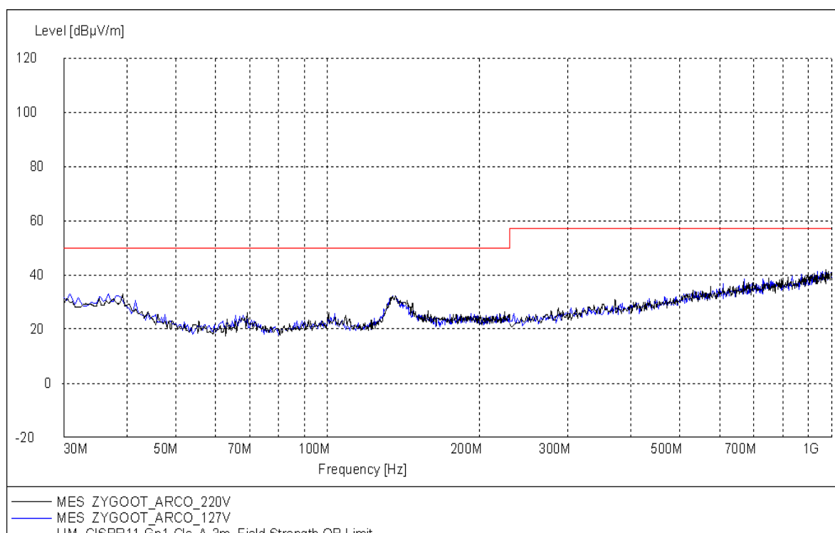
Gráfico 2 - Prévia do Ensaio de Emissão de Perturbação Radiada – Configuração Padrão - Alimentação 127V @ 60 Hz / 220V @ 60 Hz – Amostra 5284
