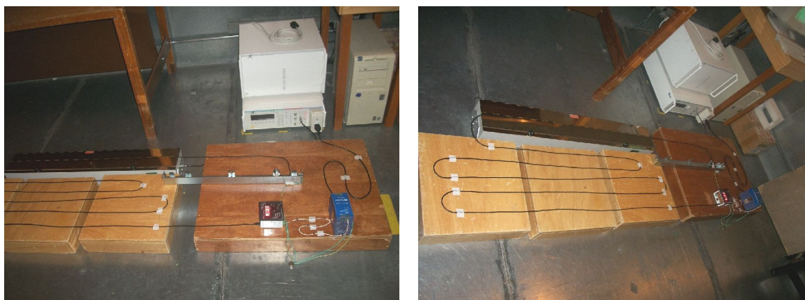
Fotos 18 e 19 – Imunidade a transientes elétricos rápidos
